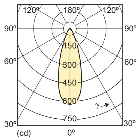
4-35W GU10 830 3000K 40D
