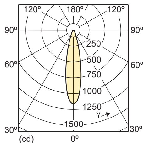
4-35W GU10 840 4000K 25D
