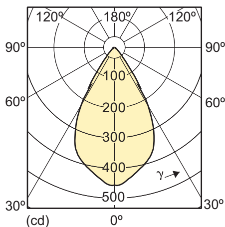
5.5-50W GU10 830 3000K 60D
