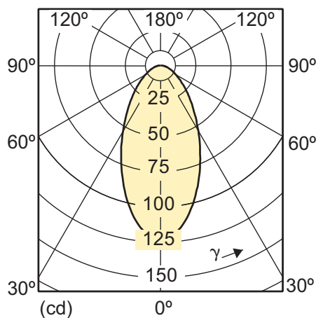
2-20W GU10 3000K 50D
