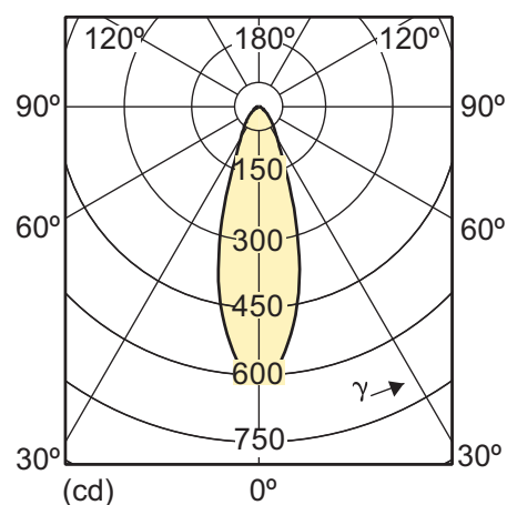
6-50W GU10 WH 40D 3000K
