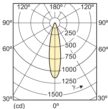
4-35W GU10 830 3000K 25D
