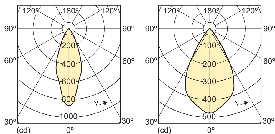
5.5-50W GU10 840 4000K 40D
