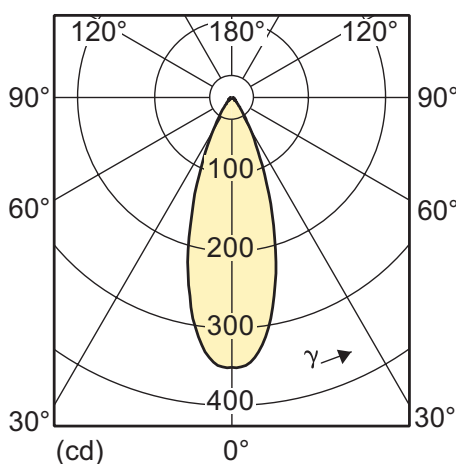
4-35W GU10 WH 40D
