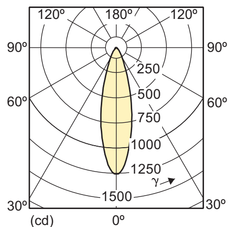
5.5-50W GU10 840 4000K 25D
