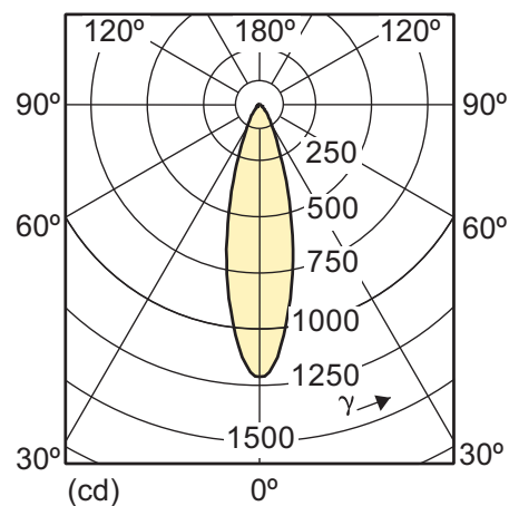
5.5-50W GU10 830 3000K 25D
