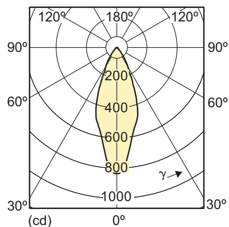
5.5-50W GU10 830 3000K 40D
