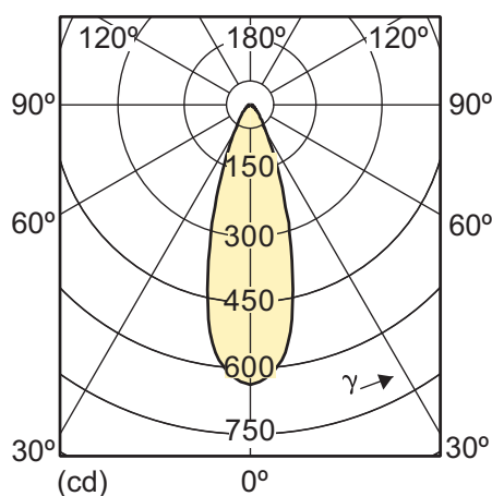
4-35W GU10 840 4000K 40D
